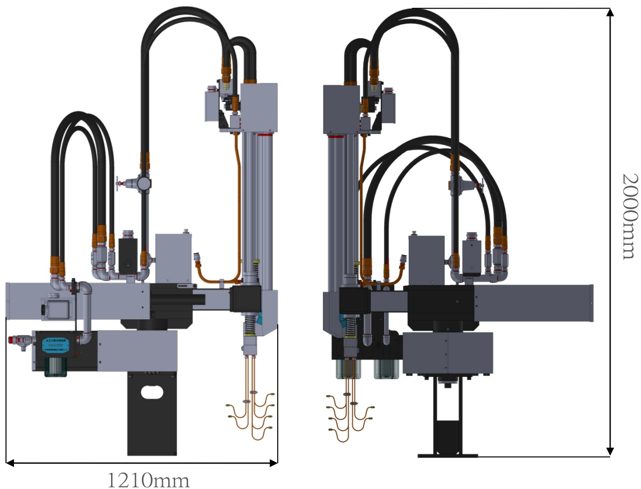
DH-D250T 直立式雙液噴霧機式樣規範
