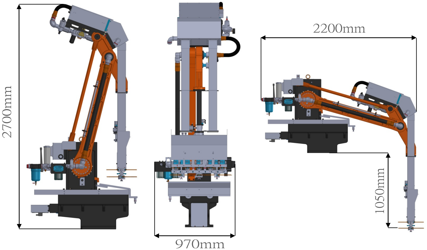
BW-D800T-BD 全控式雙液伺服噴霧機
